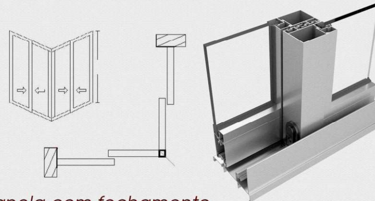
Janela com fechamento de canto
