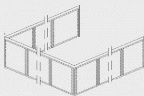
Guarda corpo de canto em vidro PANORAMA
