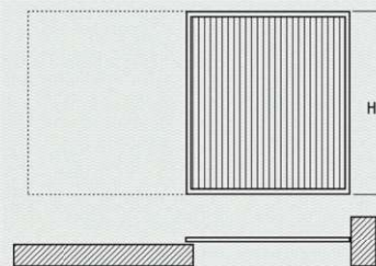
Portão de correr com 1 folha
