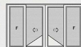
6 folhas de correr 4 venezianas e 2 vidros
